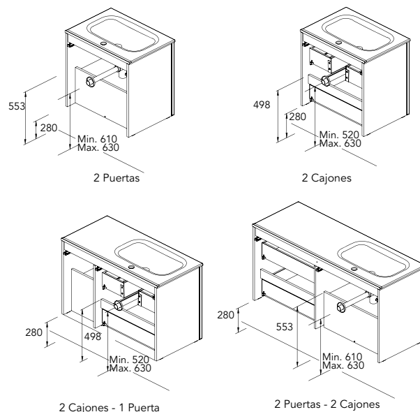
Esquema de colocación del sifón
