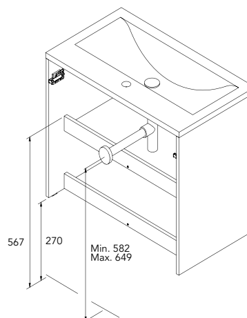
Esquema de colocación del sifón
